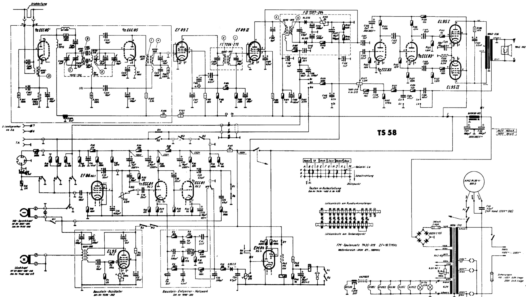
GRUNDIG WERKE - Mod. TS 58. Apparecchio radio a modulazione di frequenza, al quale è unito il registratore magnetico. Lo stadio finale funziona con il registratore o con l'apparecchio radio. Media frequenza a 10,7 Mc/s. Resa d'uscita 6 watt. Consumo 0,8 ampere a -25 volt.
